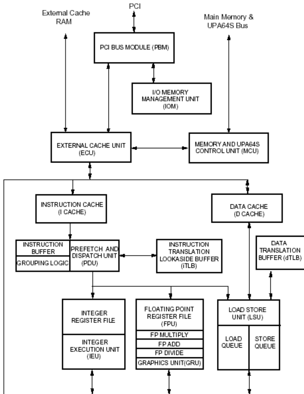
Abbildung A.1: UltraSPARC-II
