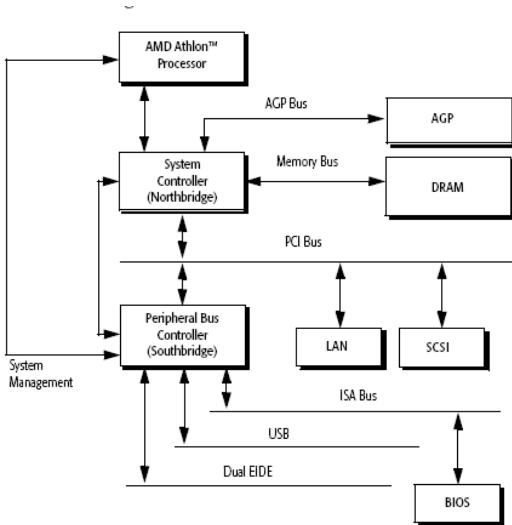
Abbildung 1.39: Athlon 32 Bit mit FSB
