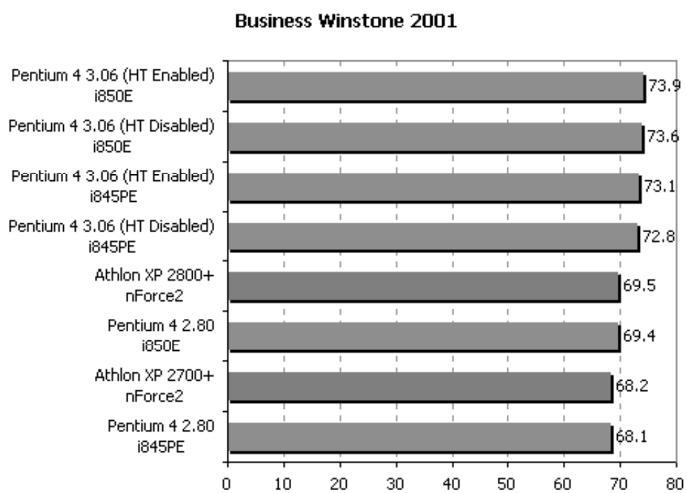
Abbildung 1.26: Hyperthreading (Fortsetzung)
