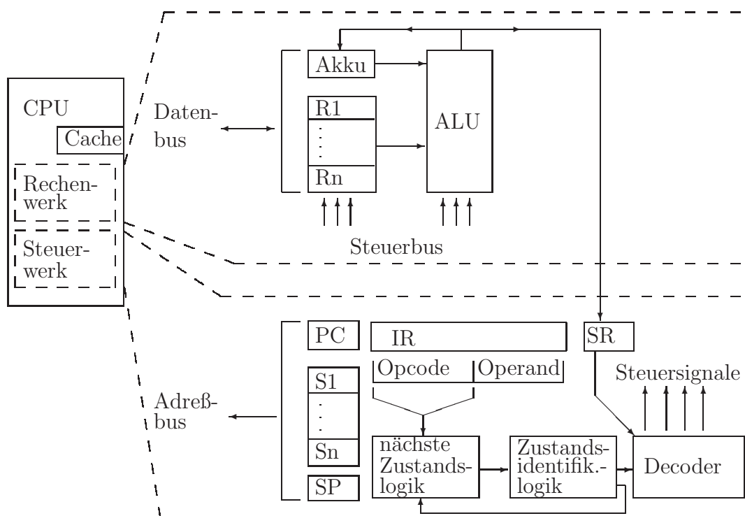
Abbildung 1.17: CISC-CPU-Aufbau
