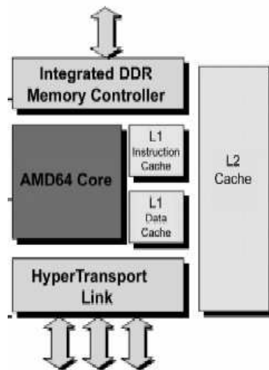
Abbildung 1.23: Alternative zum FSB: Der Opteron Hypertransport-Link
