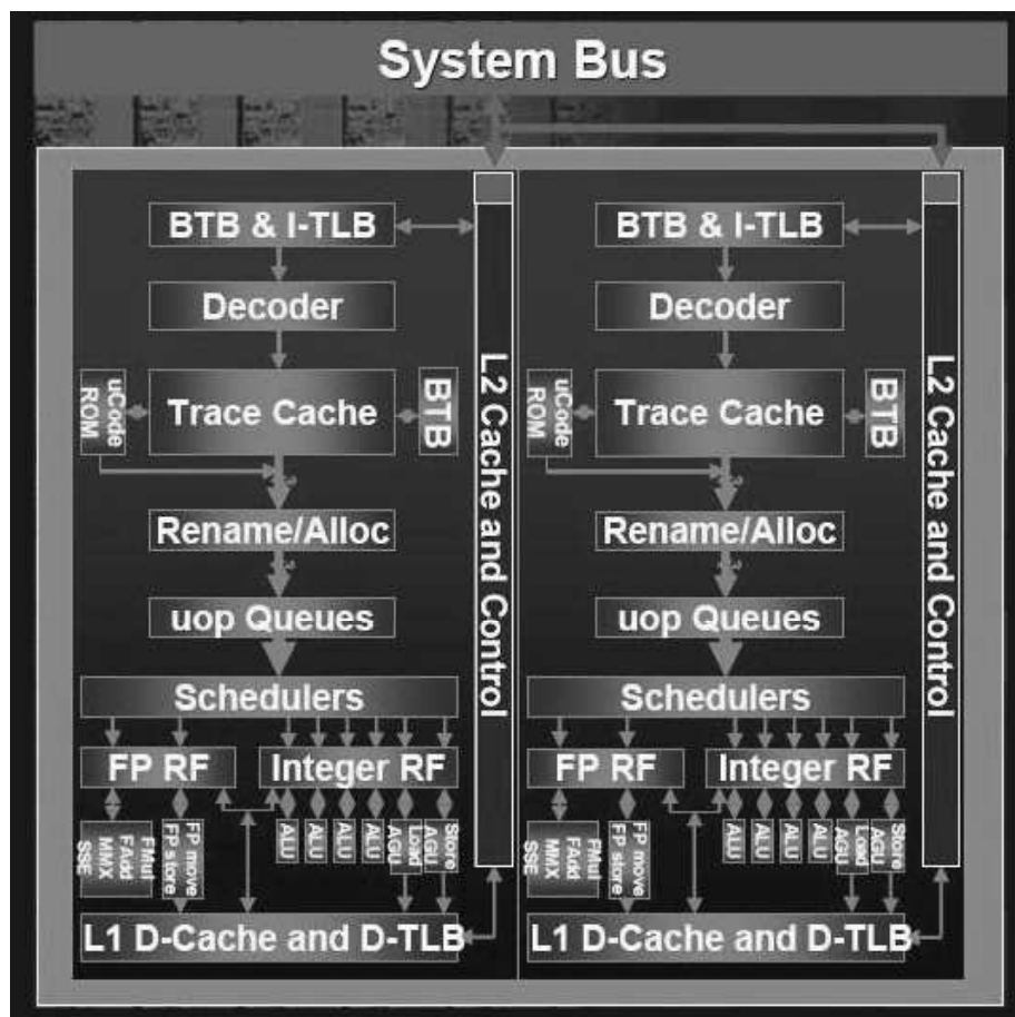
Abbildung 1.29: Dual Core Pentium D
