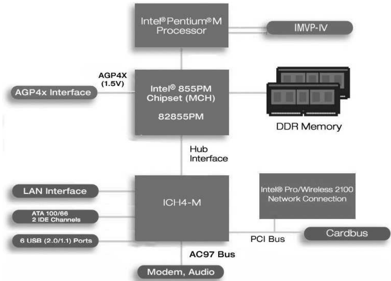
Abbildung 1.28: PentiumM
