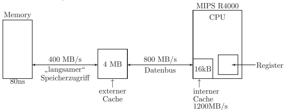
Abbildung 1.17: Der Cache als Daten-Vorratsbehälter
