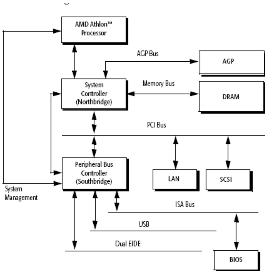
Abbildung 1.20: Athlon 32 Bit mit FSB
