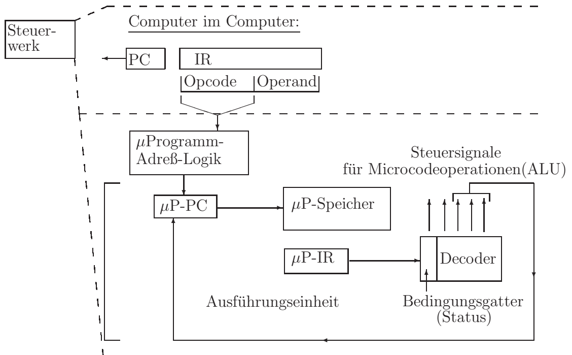
Abbildung 1.13: Microprogrammierte CISC-CPU
