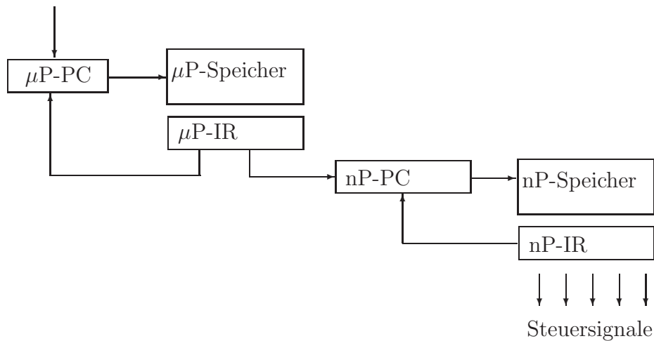
Abbildung 1.14: Nanoprogrammierte CISC-CPU
